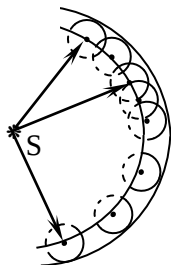
Рис. 21. Принцип Гюйгенса
