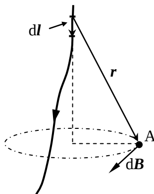
Рис.2. К закону Био-Савара – Лапласа
