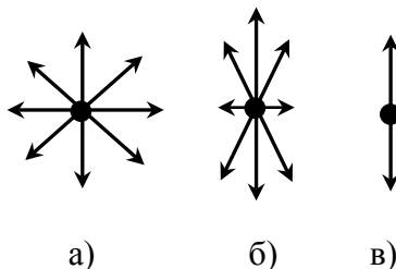
Рис.29. Виды света:
