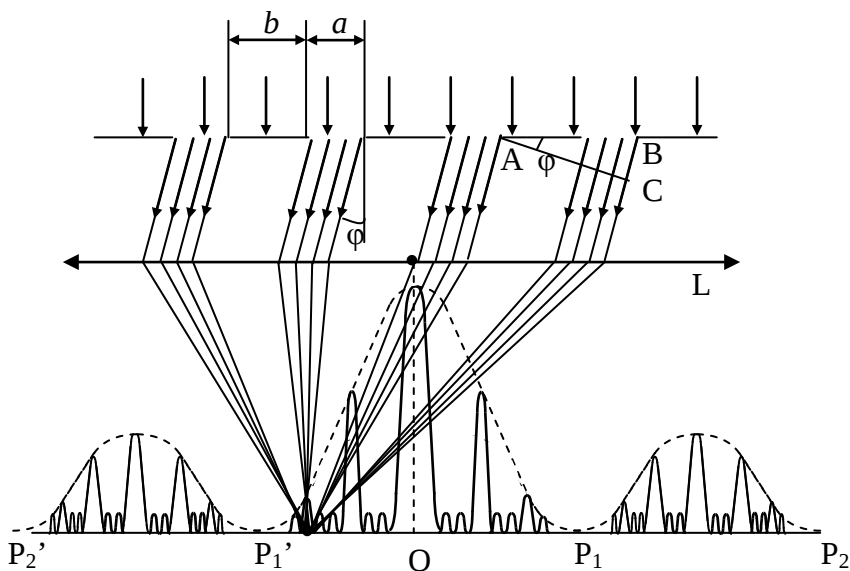
Рис. 27. Дифракция света на одномерной решетке
