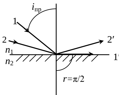
Рис. 10. Явление полного внутреннего отражения
