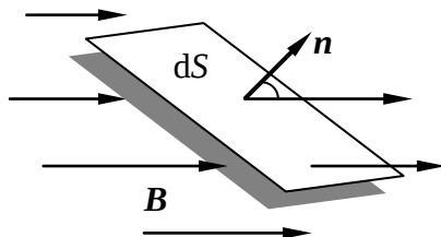
Рис.6. Определение магнитного потока
