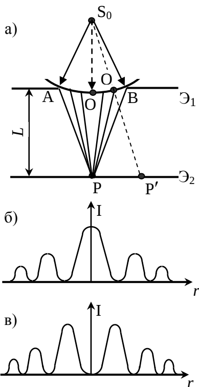
Рис. 24. а – дифракция на круглом отверстии, б – зависимость интенсивности света I от расстояния r от центра экрана для нечетного числа m ; в – для четного числа m
