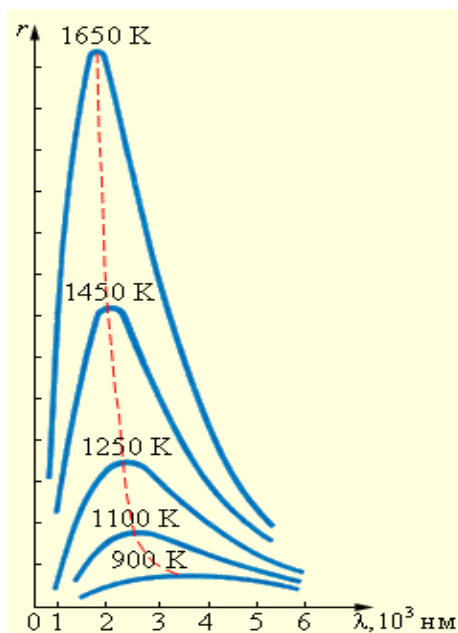
Рис. 38. Спектральное распределение излучения черного тела при различных температурах.
