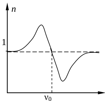
Рис. 36. Нормальная и аномальная дисперсия света в веществе
