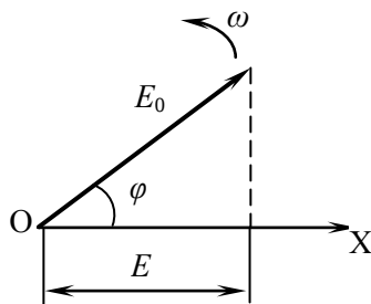
Рис.14. Метод вращающегося вектора амплитуды
