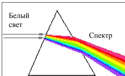
Рис. 35. Дисперсия света в стеклянной призме
