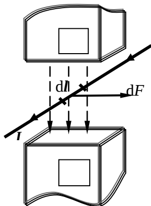
Рис.5. Сила Ампера, действующая на проводник с током в магнитном поле
