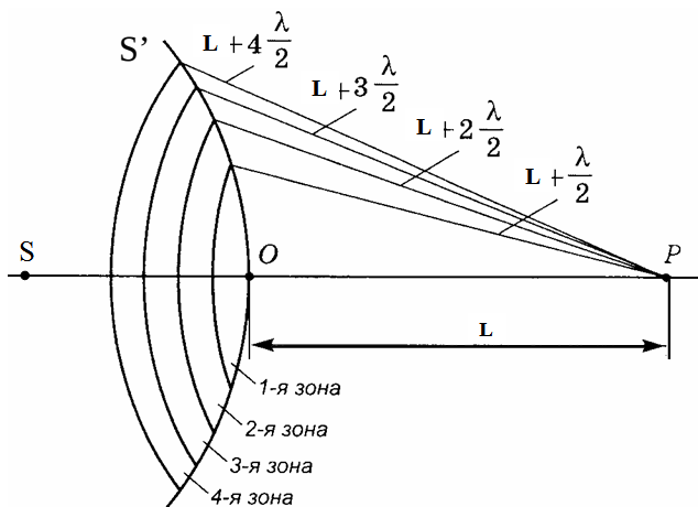
Рис. 23. Иллюстрация к методу зон Френеля
