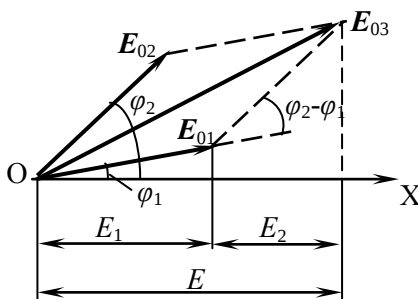
Рис. 15. Сложение гармонических колебаний
