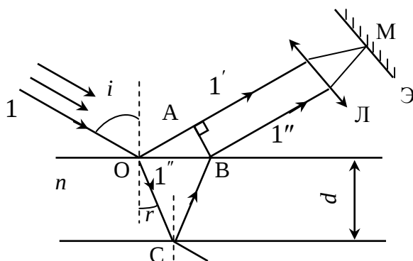
Рис. 17. Интерференция света в плоскопараллельной пленке
