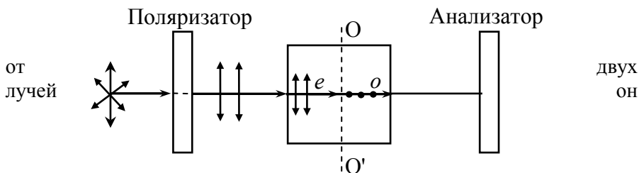
Рис. 34. Интерференция поляризованного света
