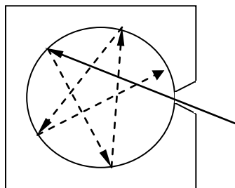
Рис.37. Модель абсолютно черного тела
