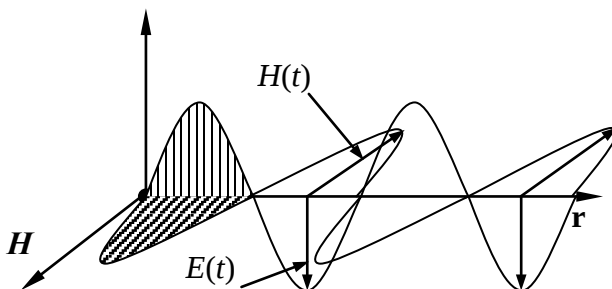
Рис. 12. Электромагнитная волна
