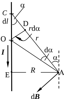
Рис.3. Магнитное поле прямолинейного проводника с током
