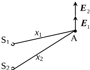
Рис. 13. Интерференция света
