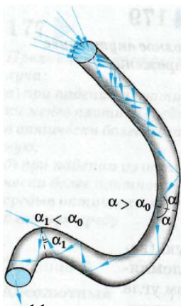
Рис. 11. Распространение света в световоде
