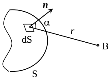
Рис. 22. Иллюстрация принципа Гюйгенса-Френеля
