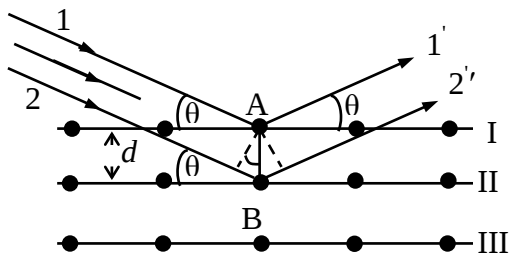
Рис. 28. К выводу формулы Вульфа – Брэгга.
