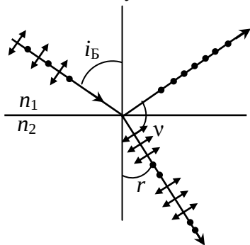
Рис. 31. Иллюстрация закона Брюстера
