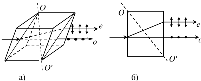
Рис. 32. а – двойное лучепреломление в кристалле. Обыкновенный и необыкновенный лучи; б – главное сечение кристалла
