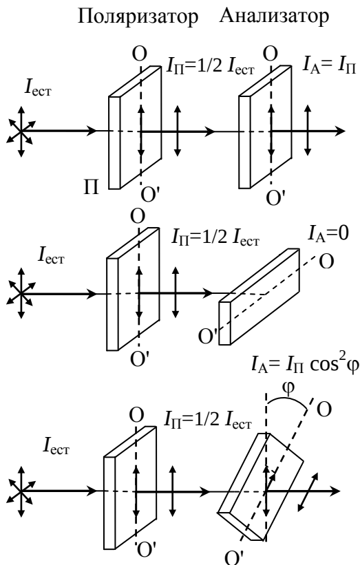
Рис. 30. Анализ поляризованного света
