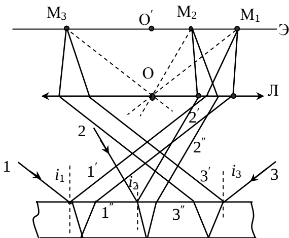
Рис. 18. Полосы равного наклона
