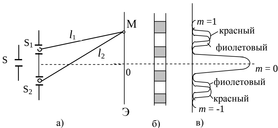
Рис. 16. Схема интерференционной картины
