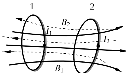
Рис.8. Явление взаимной индукции
