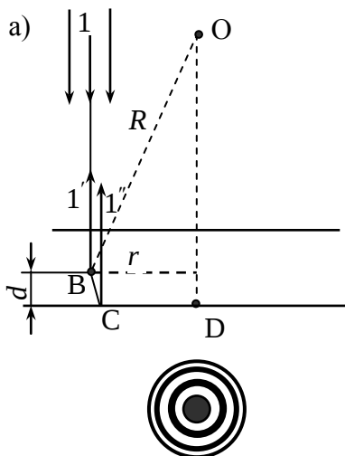
Рис. 20. Кольца Ньютона; а – оптическая схема, б – интерференционная картина
