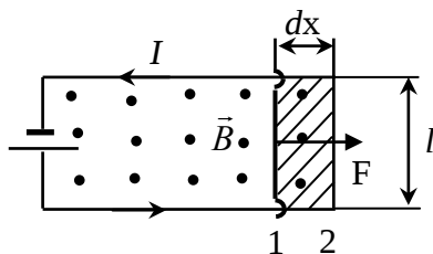
Рис.7. Проводник с током в магнитном поле
