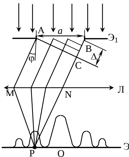
Рис. 26. Дифракция плоской волны от щели
