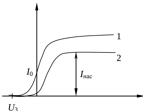
Рис. 41. Зависимости фототока I от напряжения U между электродами при различных интенсивностях падающего света E ( E_1 > E_2 ).
