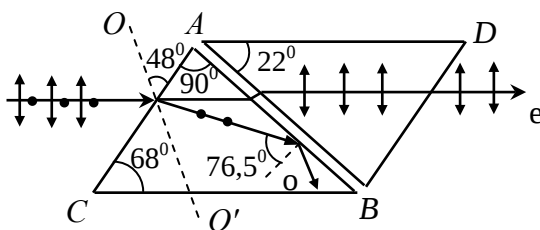
Рис.33. Призма Николя
