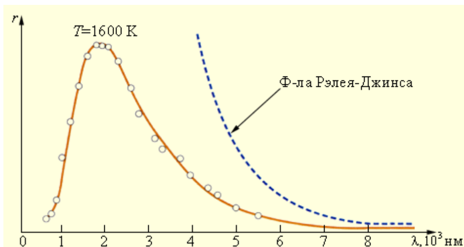
Рис. 39. Сравнение закона распределения энергии по длинам волн r(\lambda, T) в излучении абсолютно черного тела с формулой Рэлея–Джинса при T = 1600 \text{ K} .
