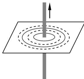
Рис.1. Силовые линии магнитного поля
