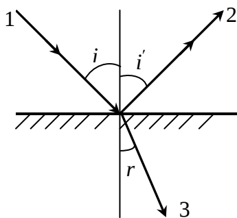
Рис. 9. Законы отражения и преломления
