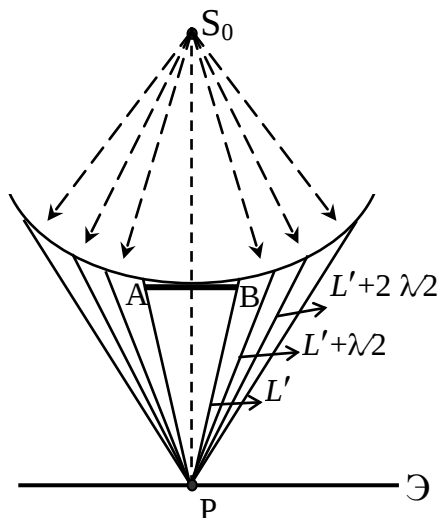
Рис. 25. Дифракция на диске
