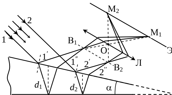
Рис.19. Интерференция света в клине
