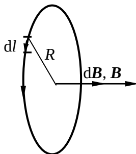
Рис.4. Магнитное поле в центре кругового проводника с током
