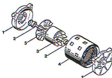
Рис. 1. Устройство асинхронного двигателя
