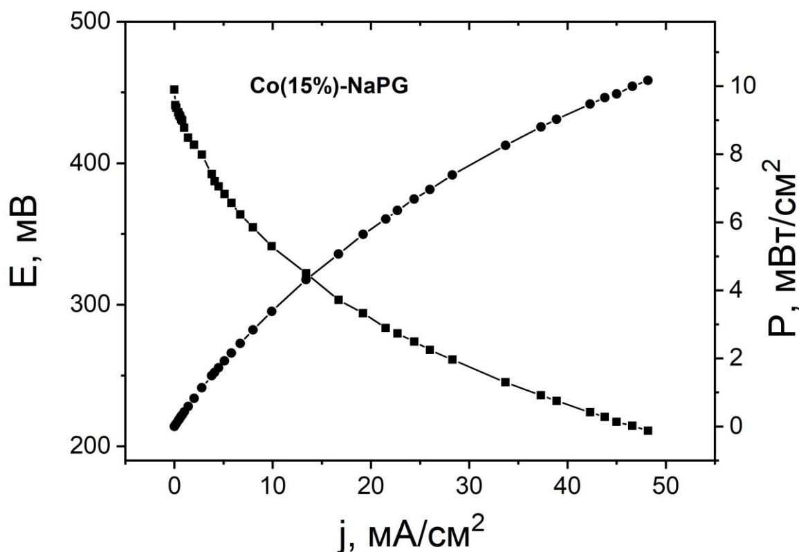
Рисунок 3.13 – Диагностические характеристики мембранно-электродного блока Pt/C/Nf/Co(15%)-NaPG/C в составе протонообменного мембранного топливного элемента: поляризационная кривая (черные квадраты); кривая зависимости плотности мощности от плотности тока (черные круги)
