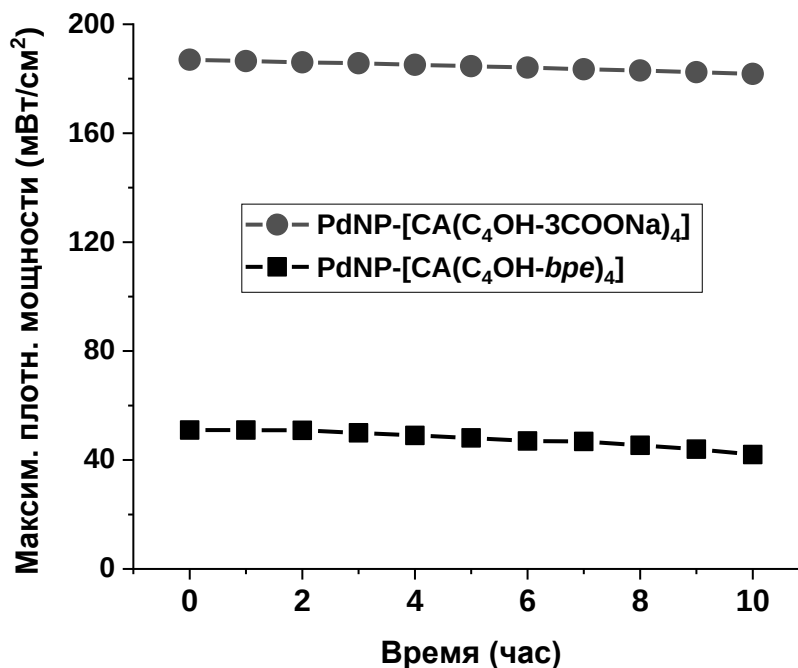
Рисунок 4.16 – Зависимость плотности мощности исследованных катализаторов PdNP-[CA(C 4 OH-3COONa) 4 ] и PdNP-[CA(C 4 OH- bpe ) 4 ] от времени работы ПОМТЭ
