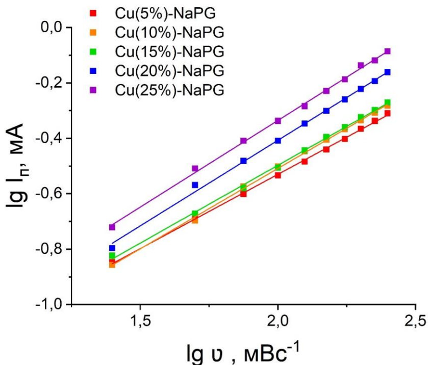
Рисунок 3.4 – Зависимости логарифма пикового тока \lg I_p от логарифма скорости развертки \lg v (25-250 мВ/с) для Cu(n%)-NaPG
