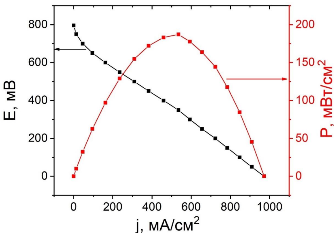
Рисунок 4.12 – Поляризационная кривая и кривая зависимости плотности мощности от плотности тока ПОМТЭ с МЭБ Pt-C/Nf/PdNP-[CA(C 4 OH-3COONa) 4 ]
