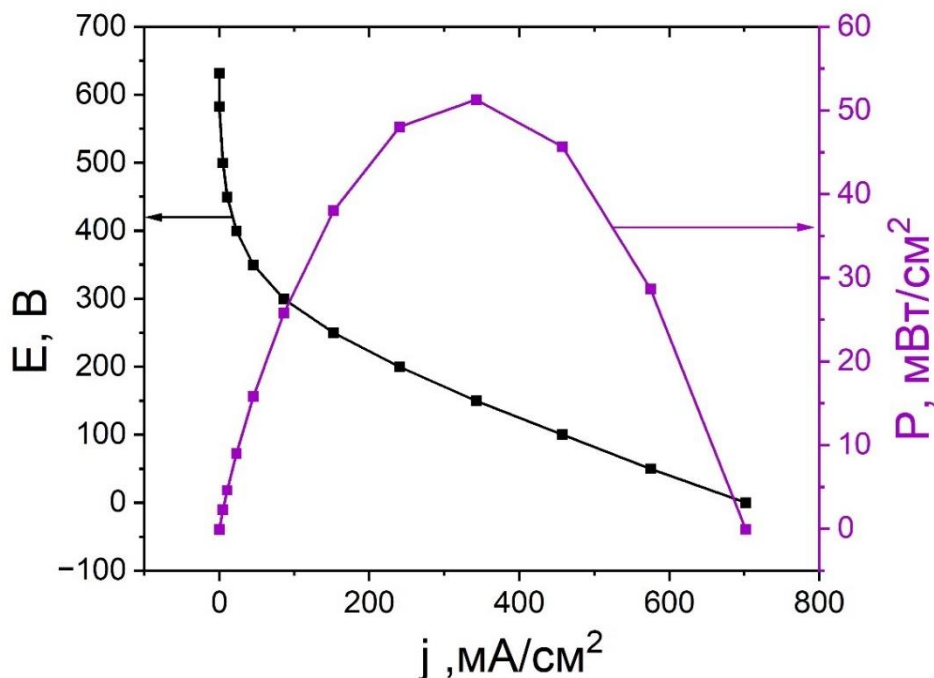
Рисунок 4.13 – Поляризационная кривая и кривая зависимости плотности мощности от плотности тока ПОМТЭ с МЭБ Pt-C/Nf/PdNP-[CA(C 4 OH-bpe) 4 ]
