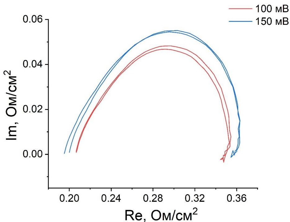
Рисунок 4.15 – Импедансы при развертке частоты от 1 Гц до 50 кГц ПОМТЭ Pt-C/Nf/PdNP-[CA(C 4 OH-bpe) 4 ] при температуре 80 °C и напряжениях 100 и 150 мВ
