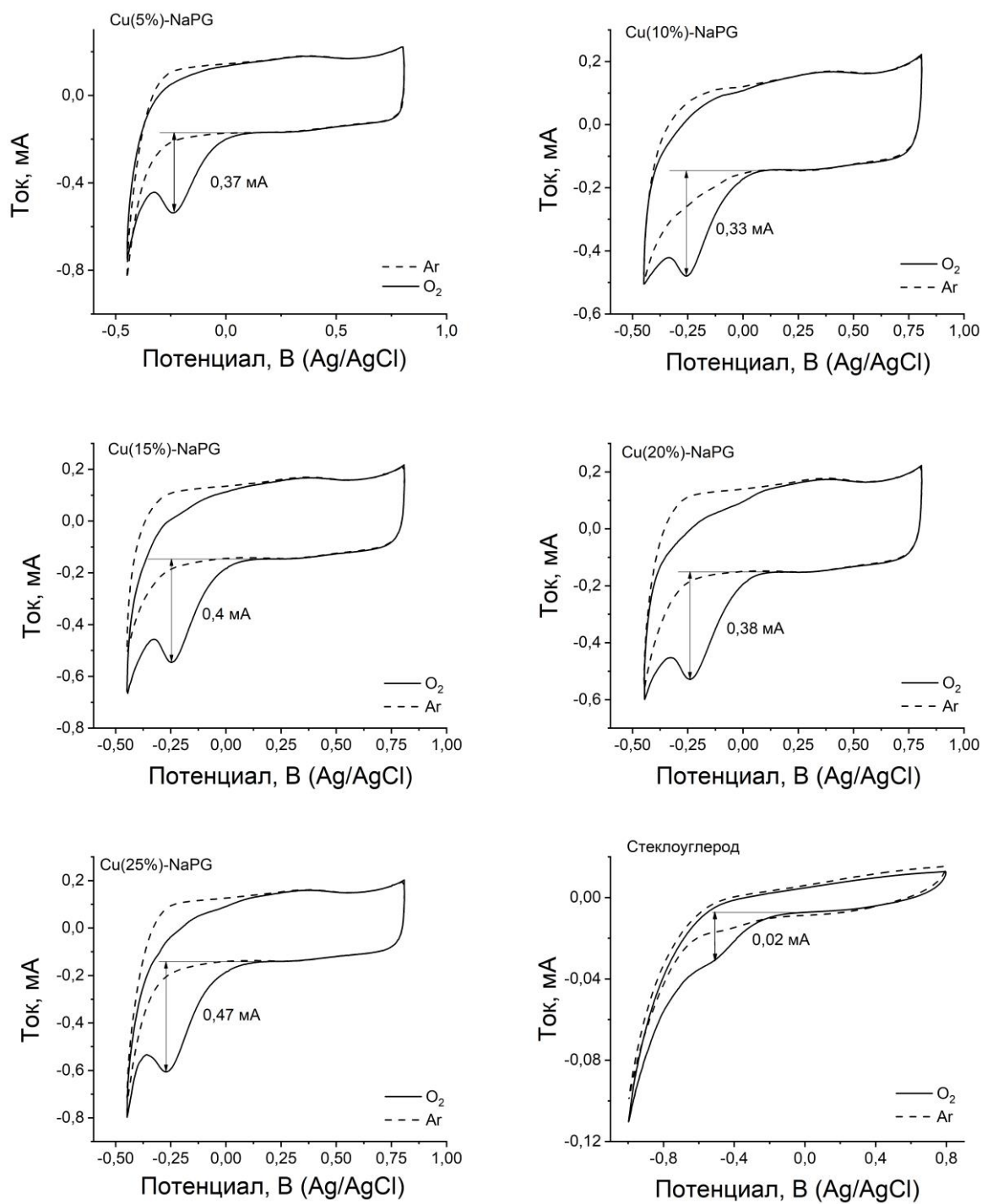
Рисунок 3.2 – ЦВА-кривые композиций Cu(n%)-NaPG в среде 0,5 М H 2 SO 4 , насыщенном O 2 и Ar, при скорости сканирования 50 мВ/с
