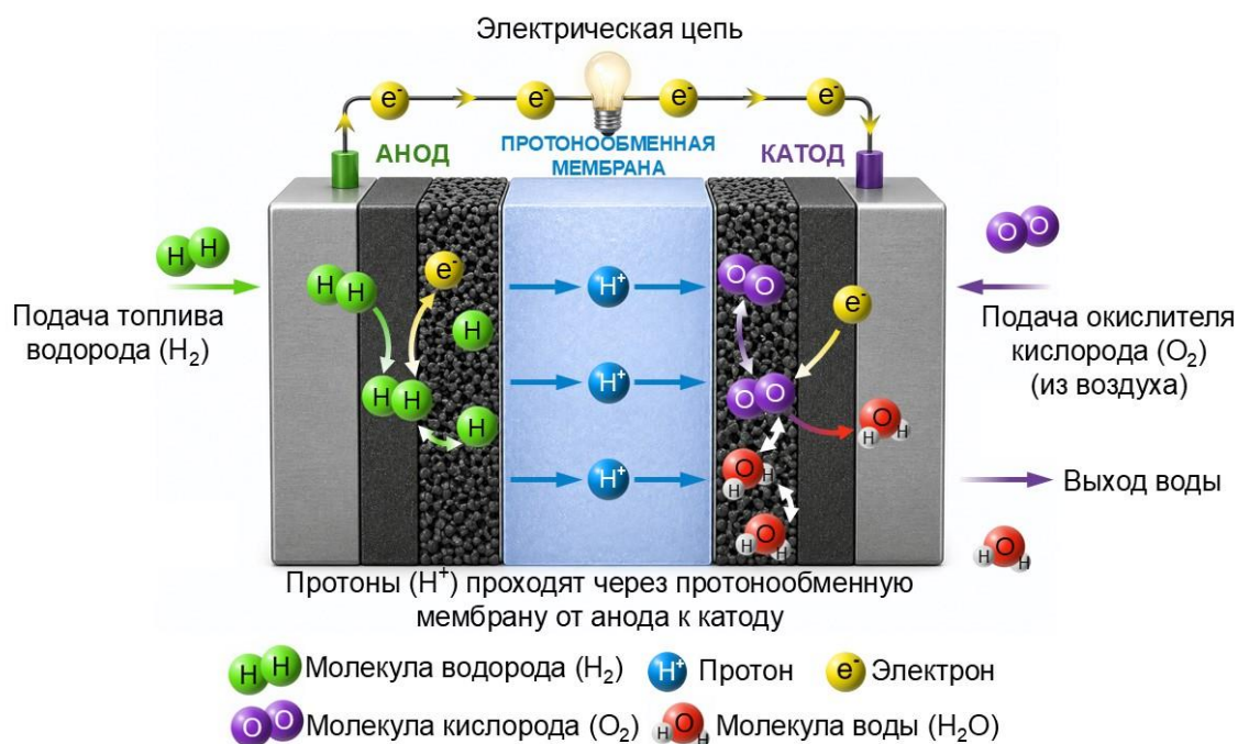
Рисунок 1.1 – Схематичное представление ПОМТЭ
