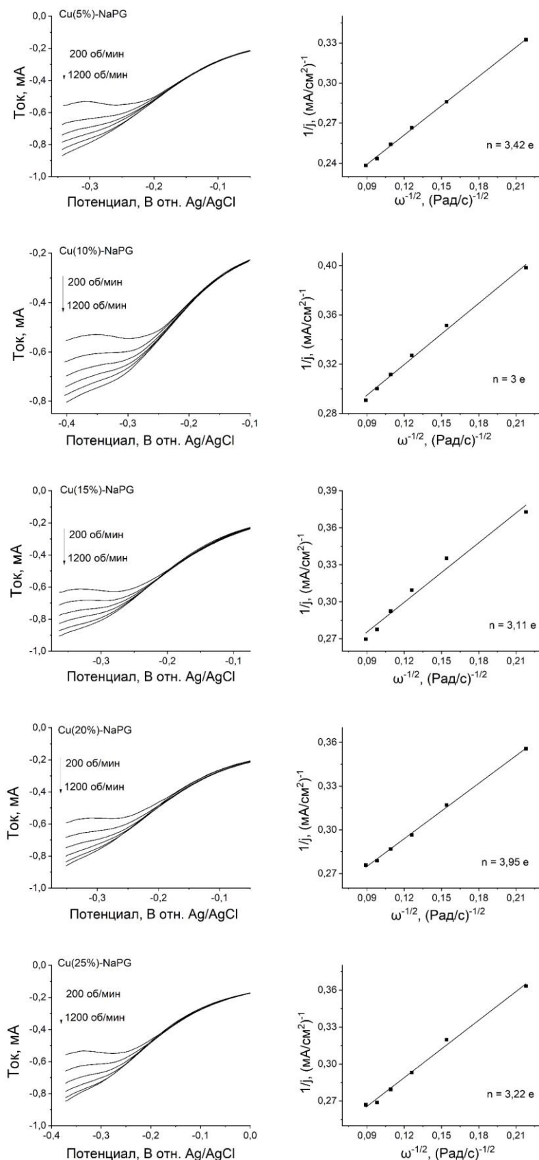
Рисунок 3.7 – ЛВА - кривые катализаторов на основе Cu(n%)-NaPG, полученные при различных скоростях вращения электрода (левый столбец); соответствующие зависимости Коутецкого-Левича (правый столбец)
