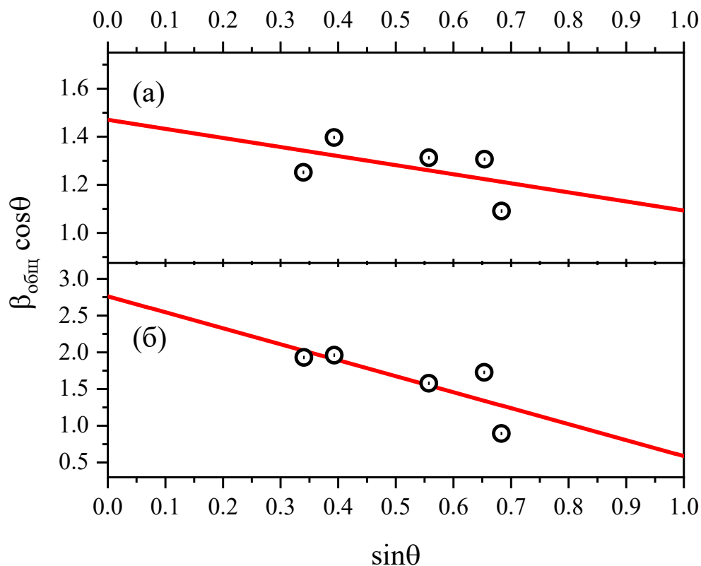
Рисунок 4.7 – Графики Уильямсона-Холла для рефлексов, связанных с наночастицами Pd и определенных на рентгеновских дифрактограммах образцов PdNP-[CA(C 4 OH-3COONa) 4 ] (a) и PdNP-[CA(C 4 OH-bpe) 4 ] (б)
