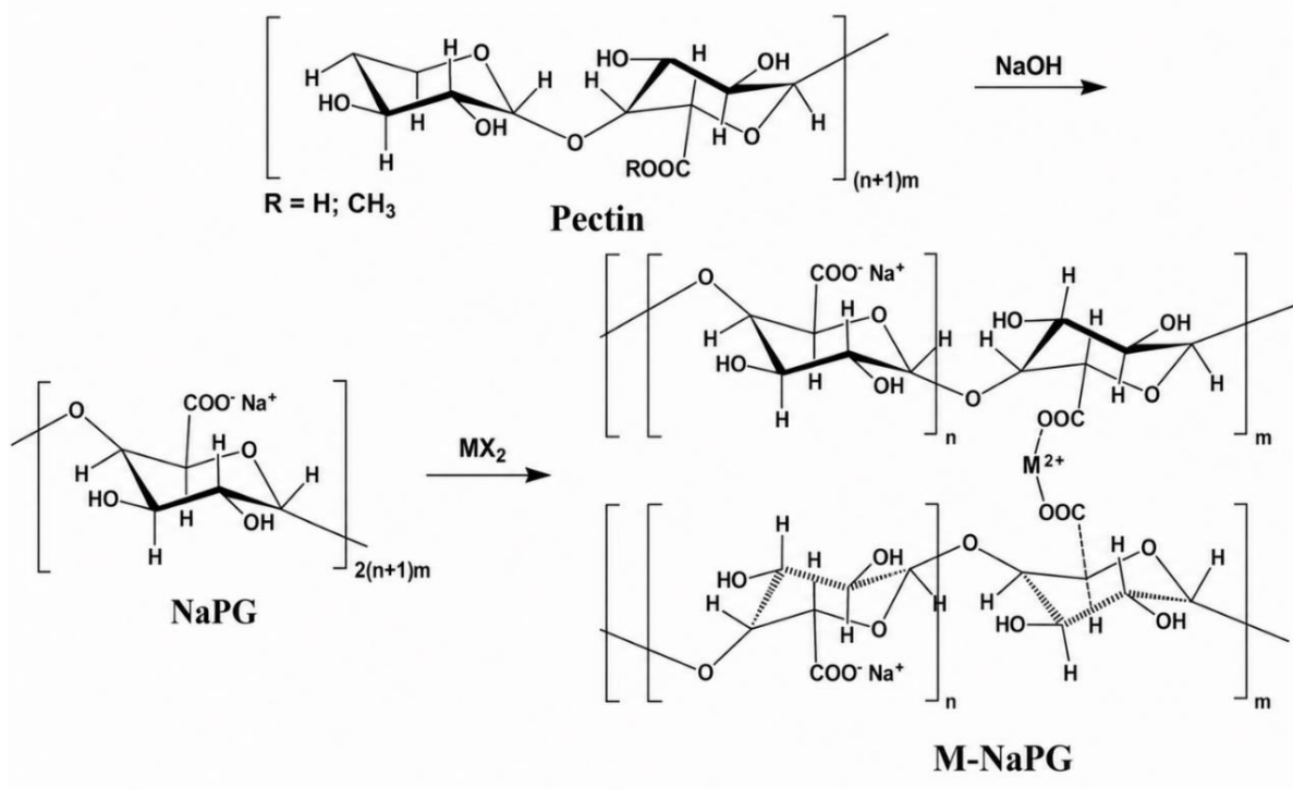
Схема 3.1 – Структура и синтез медных пектатных композиций
