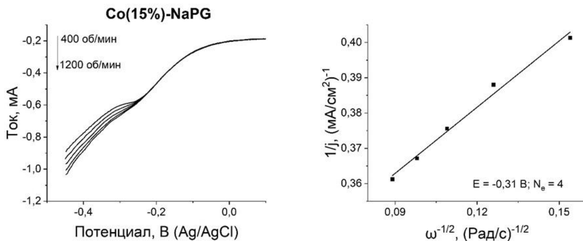
Рисунок 3.12 – Кривые линейной вольтамперометрии Co(15%)-NaPG в водном растворе 0,5 М \text{H}_2\text{SO}_4 , полученные при различных скоростях ВДЭ (слева) и зависимость Коутецкого-Левича для РВК (справа). Скорость развертки потенциала - 50 мВ/с
