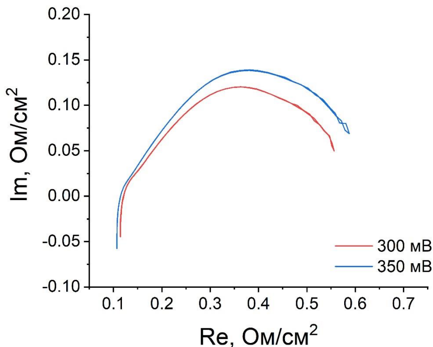
Рисунок 4.14 – Импедансы при развертке частоты от 1 Гц до 50 кГц ПОМТЭ Pt-C/Nf/PdNP- [\text{CA}(\text{C}_4\text{OH}-3\text{COONa})_4] при температуре 80 °С и напряжениях 300 и 350 мВ
