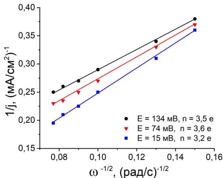
Рисунок 4.11 – Количество электронов n в РВК для катализатора PdNP-[CA(C 4 OH-3COONa) 4 ]
