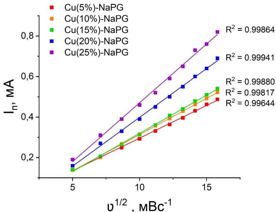
Рисунок 3.3 – Зависимости катодного пикового тока I_n от квадратного корня скорости сканирования v^{1/2} (25-250 мВ/с) для всей серии образцов Cu(n%)-NaPG
