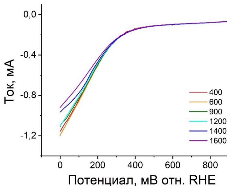
Рисунок 4.10 – Кривые ЛВА для катализатора PdNP-[CA(C 4 OH-bpe) 4 ] при восстановлении O 2
