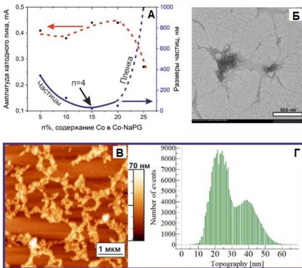
Рисунок 3.14 – Морфологические характеристики и амплитуды пика восстановления кислорода на кривых ЦВА образцов \text{Co}(n\%)\text{-NaPG} от содержания кобальта (А); ПЭМ (Б) и АСМ (В) изображения агрегатов \text{Co-NaPG} с содержанием кобальта 15% и соответствующая АСМ-изображению топографическая гистограмма (Г)
