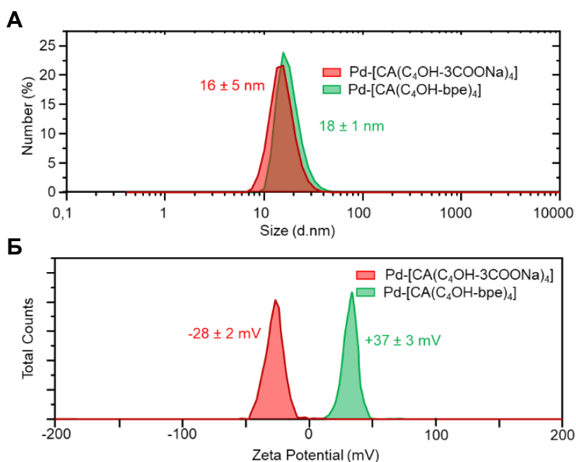
Рисунок 4.3 – Для композиций PdNP-[CA(C 4 OH-3COONa) 4 ] и PdNP-[CA(C 4 OH-bpe) 4 ]: (А) Распределение частиц по размерам по данным ДРС и (Б) Распределение ζ-потенциала, C[Pd] = 2,5 мМ, C(CA) = 0,5 мМ, H 2 O, 25°C
