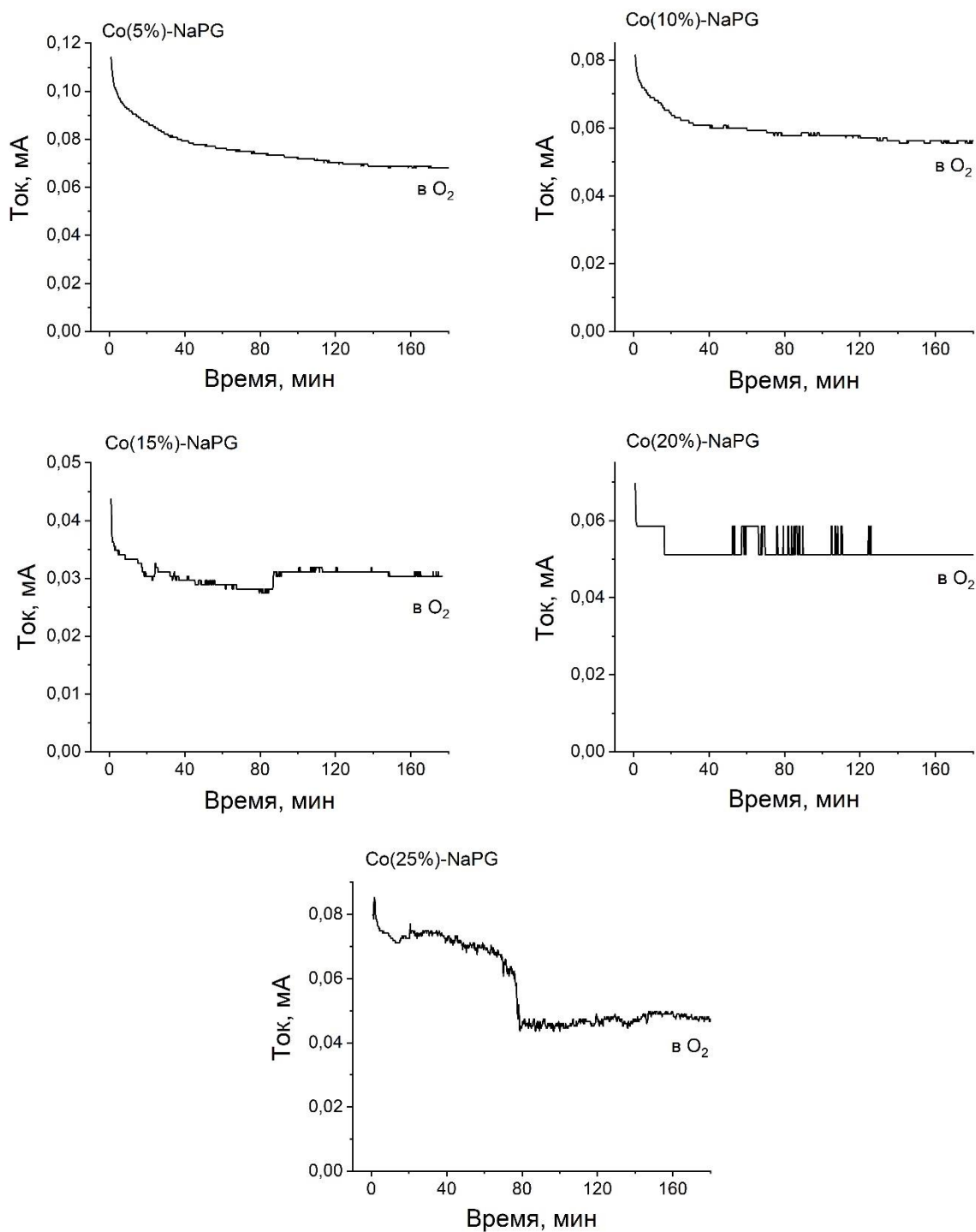
Рисунок 3.11 – Потенциостатическая стабильность кобальтовых пектатных композиций Co(n%)-NaPG в течение 3 ч в атмосфере кислорода
