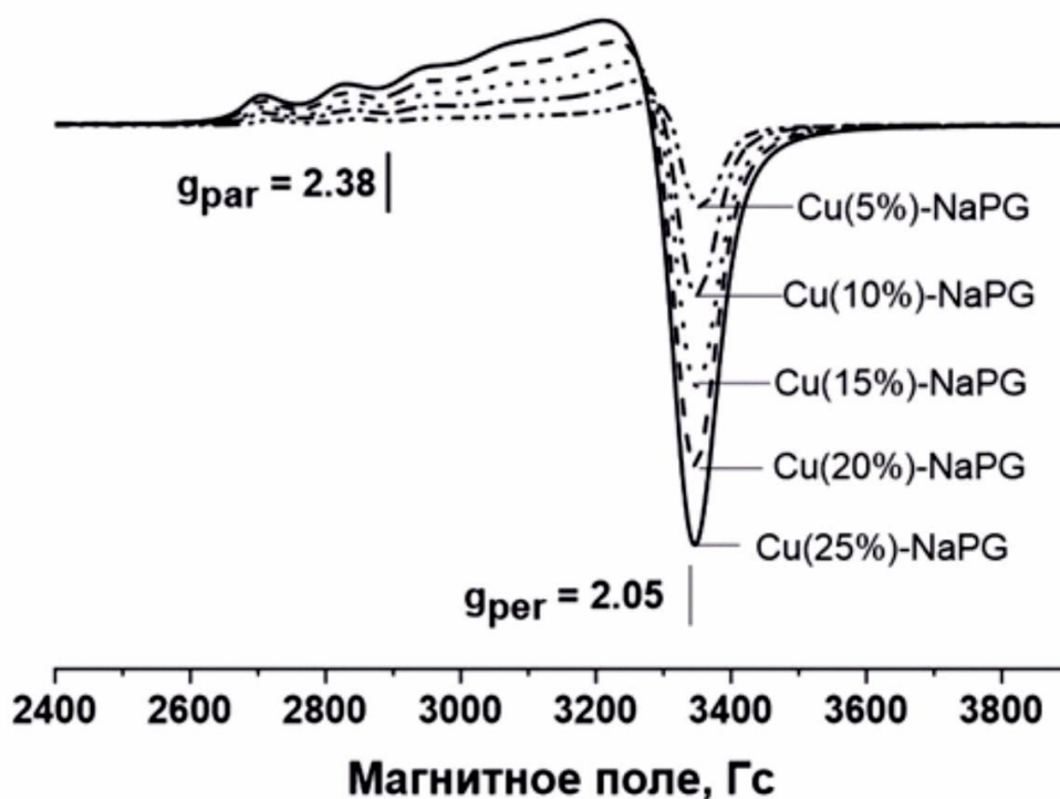
Рисунок 3.1 – Спектры ЭПР медных пектатных композиций \text{Cu}(n\text{‰})\text{-NaPG} при разных концентрациях иона меди
