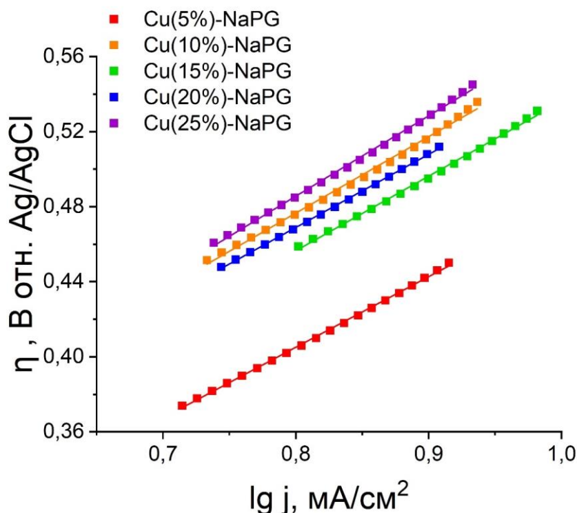
Рисунок 3.5 – Кривые Тафеля для композиций Cu(n%)-NaPG при скорости сканирования 50 мВ/с
