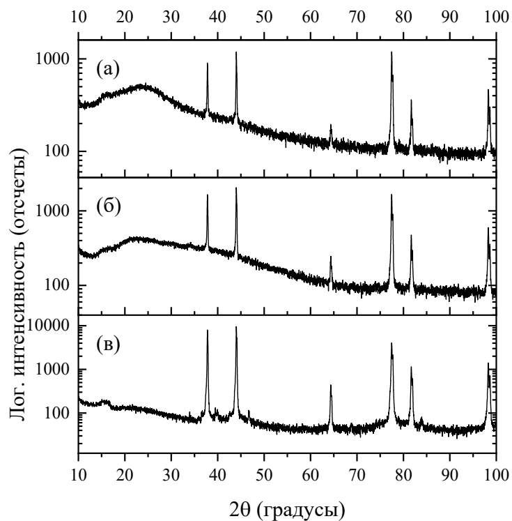
Рисунок 4.5 – Рентгеновские дифрактограммы \text{SA}(\text{C}_4\text{OH-bpe})_4 (а), \text{SA}(\text{C}_4\text{OH-3COONa})_4 (б) и алюминиевой подложки (в)
