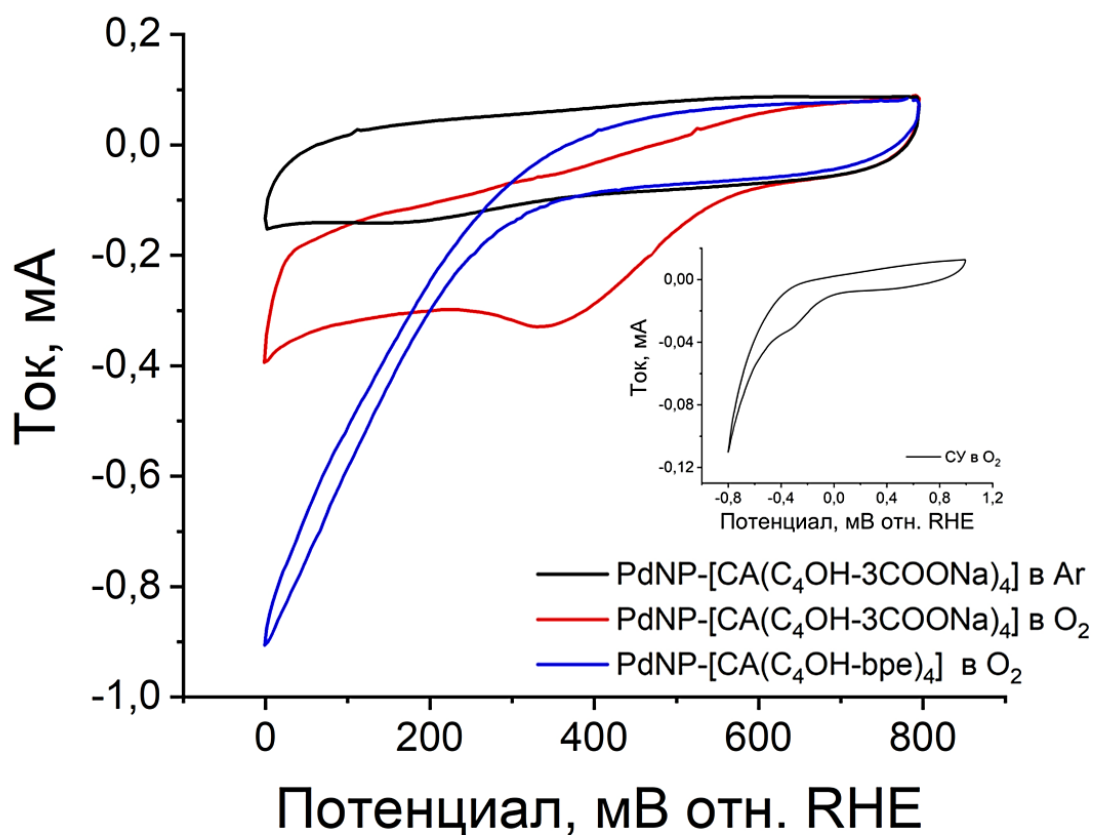
Рисунок 4.8 – ЦВА-кривые катализаторов PdNP-[CA(C 4 OH-ZCOONa) 4 ] и PdNP-[CA(C 4 OH-bpe) 4 ] в атмосфере O 2 и Ar; (вставка) – ЦВА кривая для СУ в O 2
