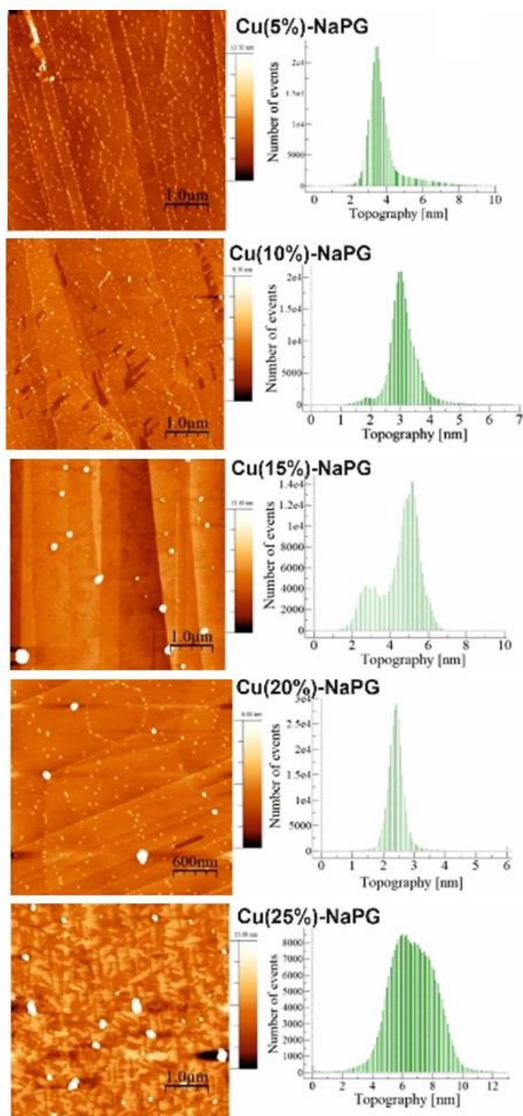
Рисунок 3.9 – АСМ изображения (левые столбцы) и топографические гистограммы (правые столбцы) катализаторов Cu(n%)-NaPG
