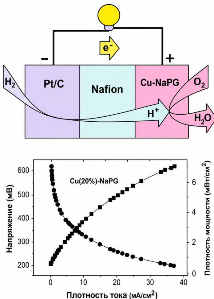
Рисунок 3.8 – Представление H 2 /O 2 Pt/C/Nf/Cu(20%)-NaPG/C ПОМТЭ (вверху); кривая поляризации (черные кружки) и кривая плотности мощности (черные квадраты) от плотности тока для Pt/C/Nf/Cu(20%)-NaPG/C ПОМТЭ
