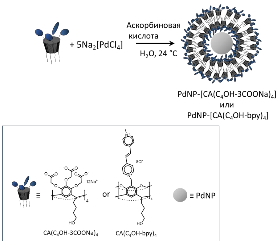
Схема 4.1 – Синтез PdNP-[CA(C 4 OH-3COONa) 4 ] и PdNP-[CA(C 4 OH-bpe) 4 ]
