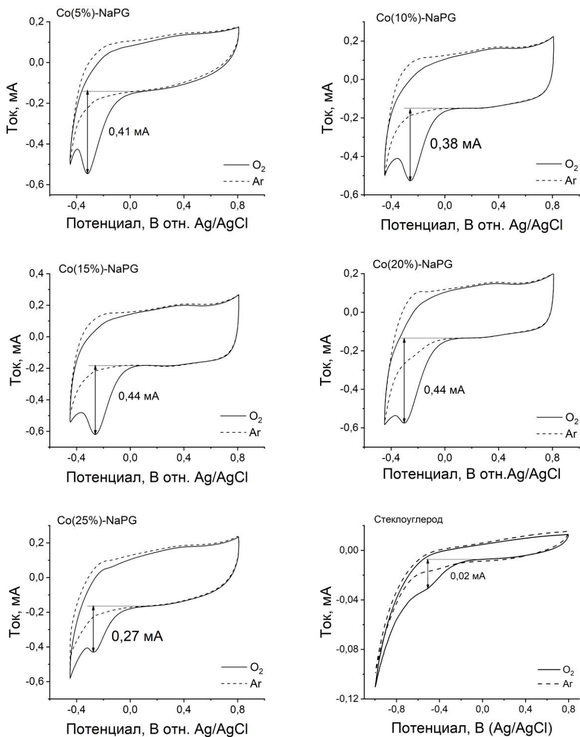
Рисунок 3.10 – ЦВА-кривые композиций Co(n%)-NaPG в среде 0,5 М H 2 SO 4 , насыщенном O 2 и Ar, при скорости сканирования 50 мВ/с
