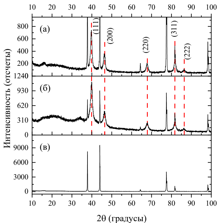
Рисунок 4.6 – Рентгеновские дифрактограммы образцов \text{PdNP}[\text{SA}(\text{C}_4\text{OH-3COONa})_4] (а) и \text{PdNP}[\text{SA}(\text{C}_4\text{OH-bpe})_4] (б), а также алюминиевой подложки (в)
