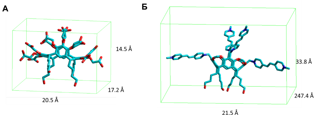
Рисунок 4.4 – Геометрические параметры молекул каликсаренов (А) CA(C 4 OH-3COONa) 4 и (Б) CA(C 4 OH-bpe) 4 , рассчитанные методом молекулярного моделирования с использованием программы HyperChem [180]
