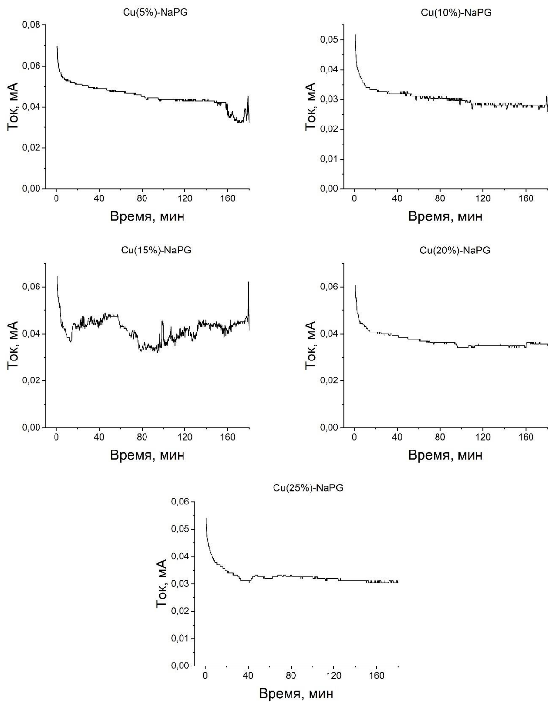
Рисунок 3.6 – Потенциостатическая стабильность медных пектатных композиций Cu(n%)-NaPG в течение 3 ч в атмосфере кислорода
