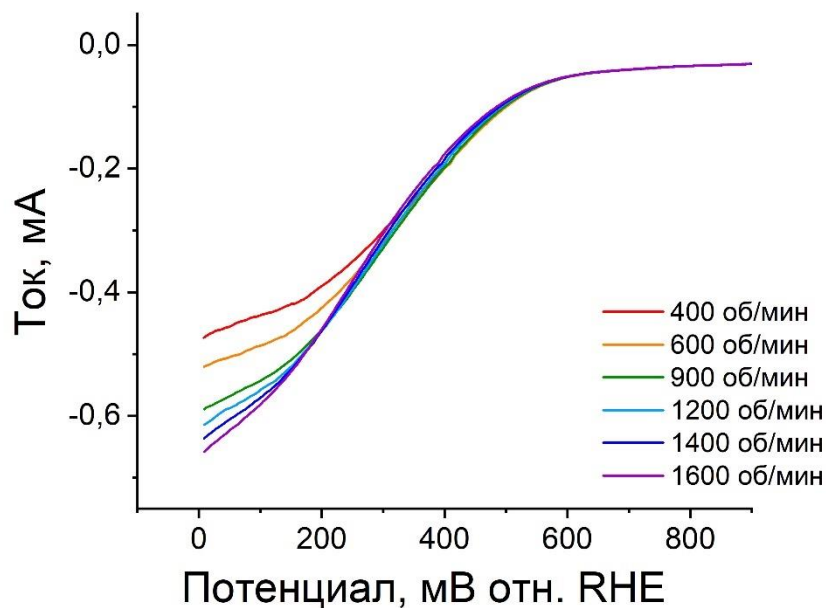
Рисунок 4.9 – Кривые ЛВА для катализатора PdNP-[CA(C 4 OH-3COONa) 4 ] при восстановлении O 2
