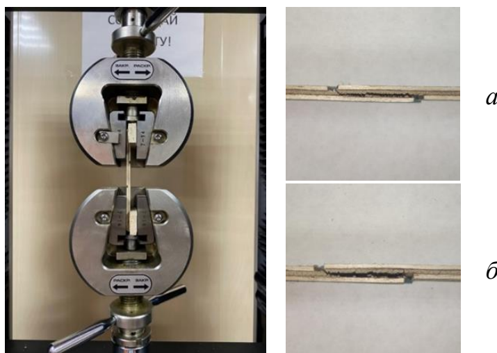
Рисунок 4.8 – Испытание образцов на сдвиг по клеевому шву: ацетилованный (а) и контрольный (б) образцы
