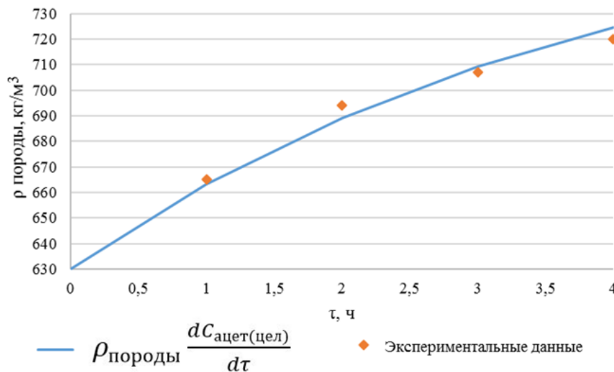
Рисунок 2.8 – Изменение плотности березы при температуре 80 °С в зависимости от продолжительности ацетилирования
