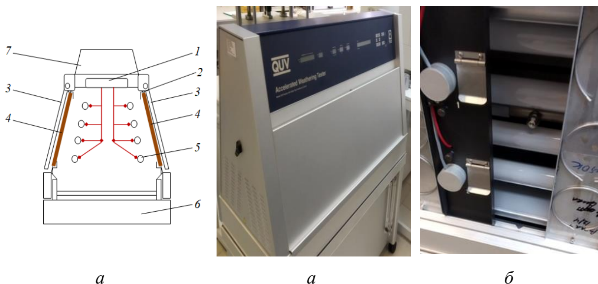
Рисунок 5.3 – Климатический стенд TSY-W3:
