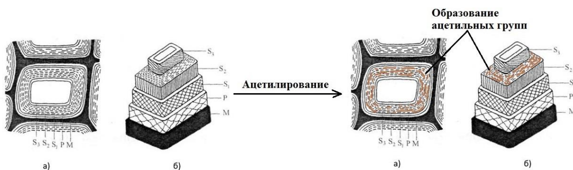
Рисунок 2.2 – Схема процесса ацетилирования:
