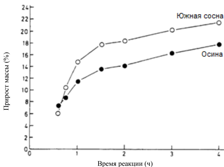
Рисунок 1.8 – Степень ацетилирования стружки южной сосны и осины в зависимости от времени реакции
