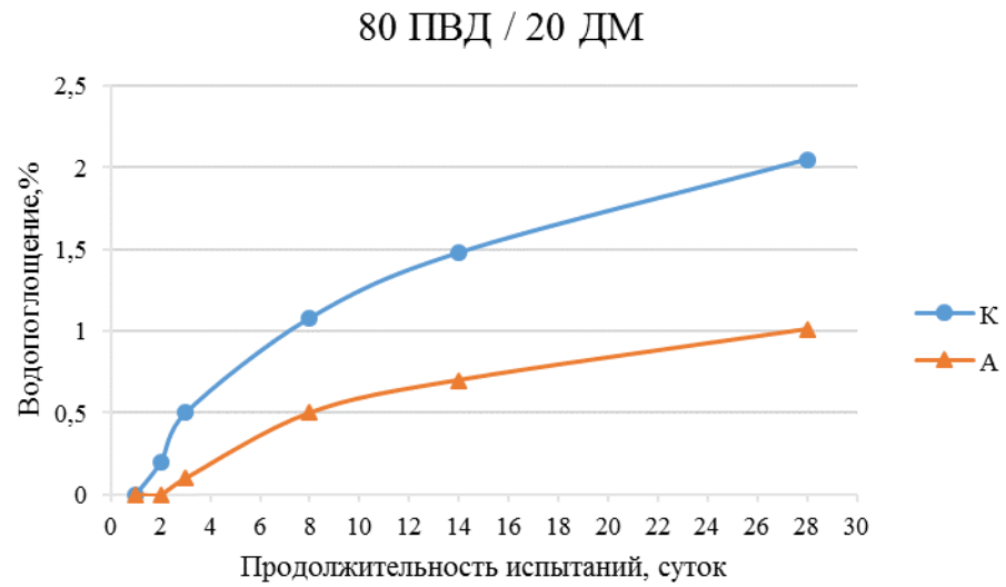
Рисунок 4.23 – Водопоглощение ДПК с 20 %-м содержанием наполнителя
