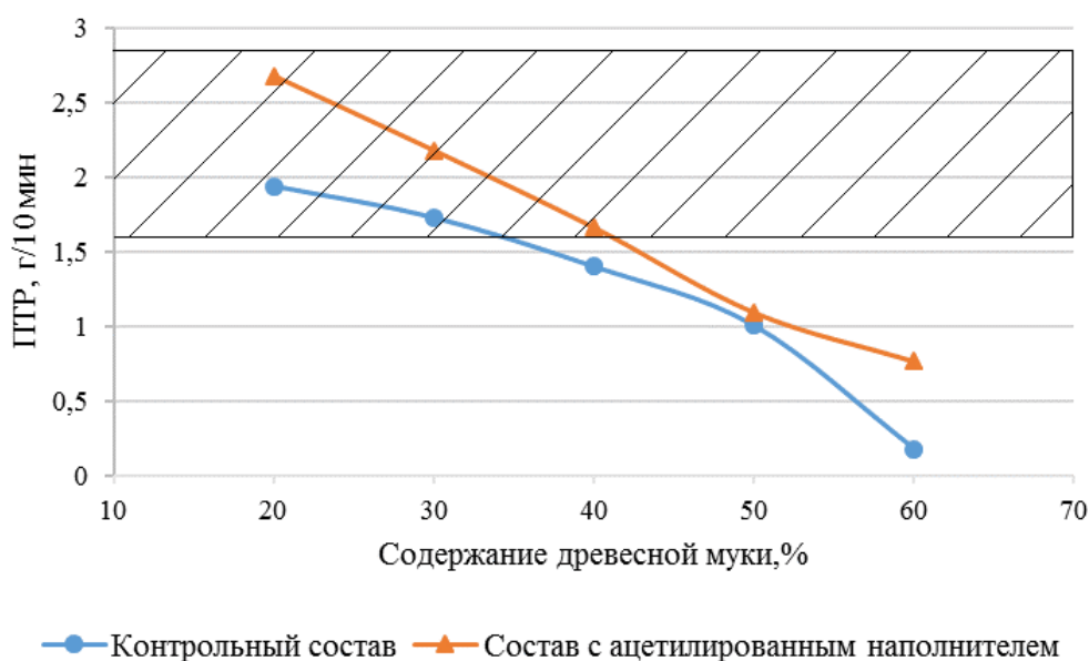
Рисунок 5.1 – Определение значений предельной текучести расплава
