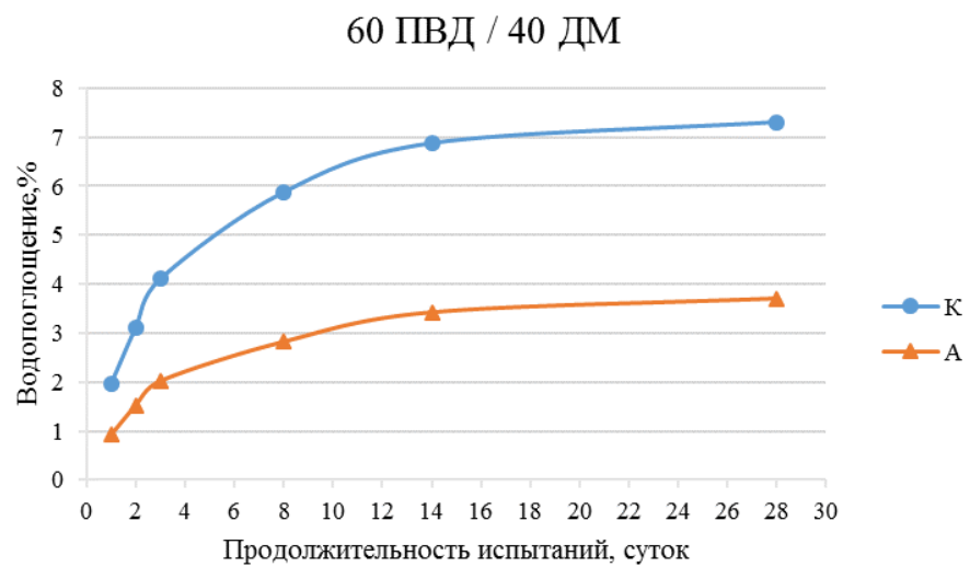
Рисунок 4.25 – Водопоглощение ДПК с 40 %-м содержанием наполнителя
