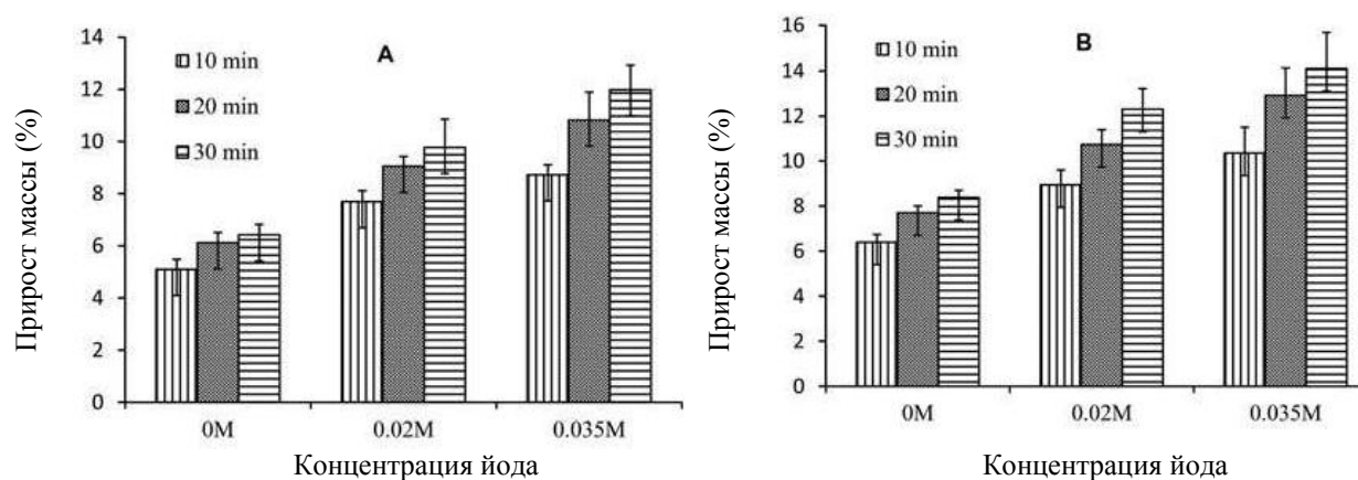
Рисунок 1.6 – Влияние микроволнового нагрева на прирост массы в присутствии уксусного ангидрида: (А) 105°C; (В) 120°C
