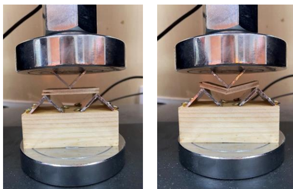
Рисунок 4.7 – Испытание образцов на прочность при изгибе
