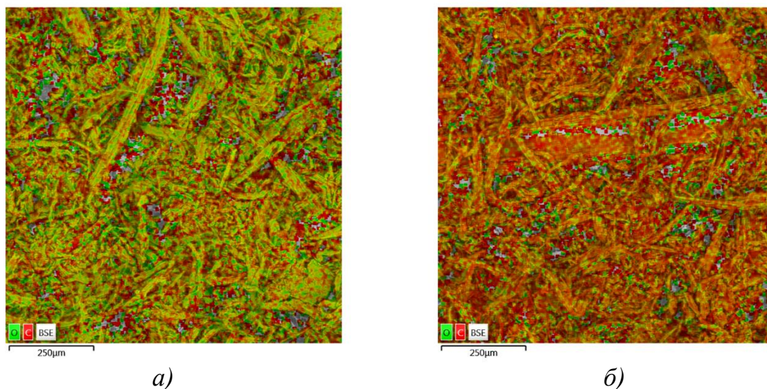
Рисунок 3.12 – Элементные карты контрольного (а) и ацетилированного (б) образцов древесной муки березы
