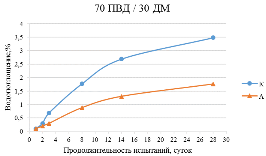
Рисунок 4.24 – Водопоглощение ДПК с 30 %-м содержанием наполнителя
