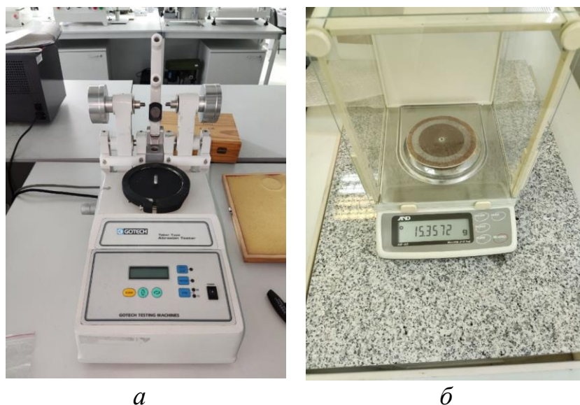
Рисунок 4.16 – Анализатор абразивный Taber GT 7012-T (а); весы лабораторные электронные HR-60 (б)
