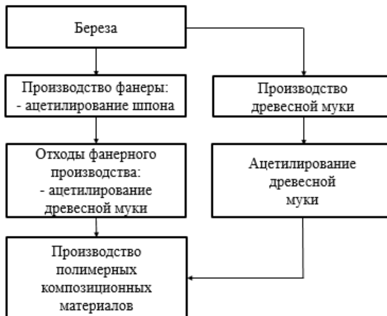
Рисунок 4.1 – Схема производства композиционных материалов
