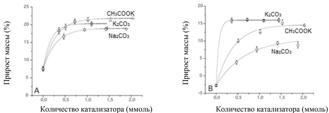
Рисунок 1.5 – Влияние типа и количества катализатора на прирост массы древесной муки, модифицированной уксусным ангидридом (А) или винилацетатом (В)
