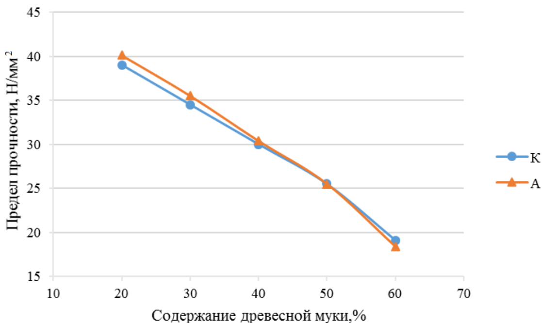
Рисунок 4.21 – Влияние концентрации и предварительной обработки контрольных (К) и ацетилированных (А) составов ДПК на предел прочности при статическом изгибе
