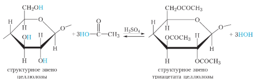
Рисунок 1.3 – Уравнение реакции структурного звена макромолекулы целлюлозы с ледяной уксусной кислотой
