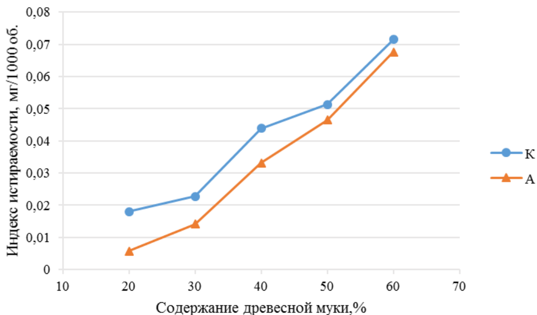
Рисунок 4.31 – Влияние концентрации и предварительной обработки контрольных (К) и ацетилированных (А) составов ДПК на индекс истираемости
