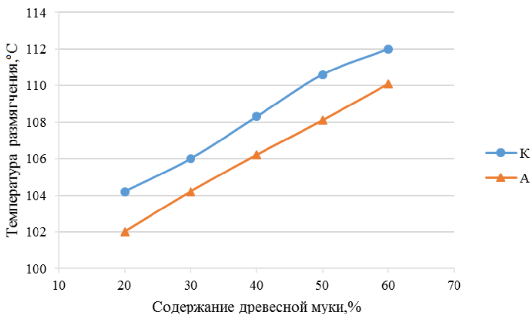
Рисунок 4.29 – Влияние концентрации и предварительной обработки контрольных (К) и ацелированных (А) составов ДПК на температуру размягчения
