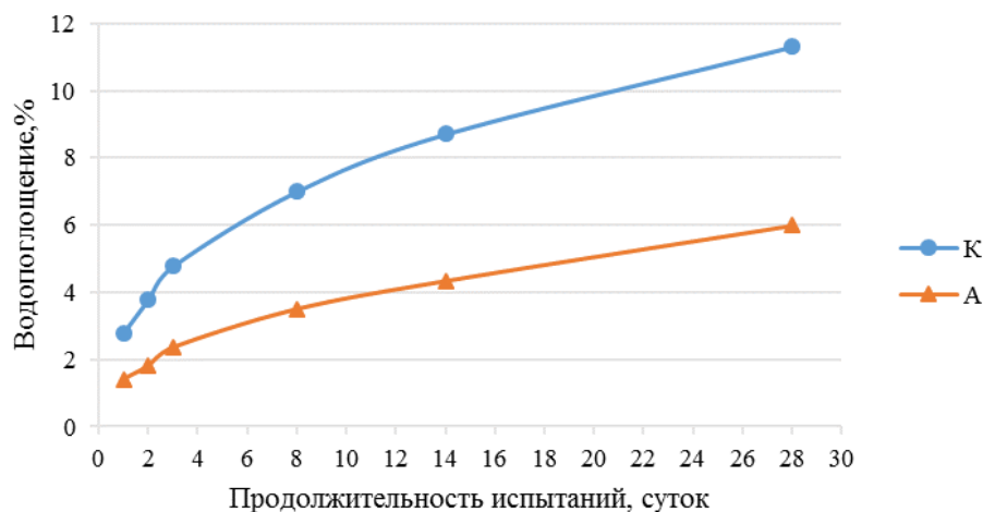
Рисунок 4.26 – Водопоглощение ДПК с 50 %-м содержанием наполнителя
