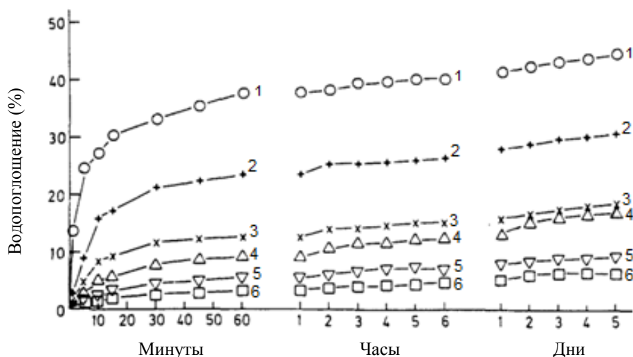
Рисунок 1.9 – Водопоглощение древесностружечных плит из южной сосны, изготовленной из ацелированных стружек: 1 – контрольный образец; 2 – прирост массы после ацелирования на 6 %; 3 – прирост массы после ацелирования на 10,4 %; 4 – прирост массы после ацелирования на 18,4 %; 5 – прирост массы после ацелирования на 21,1 %
