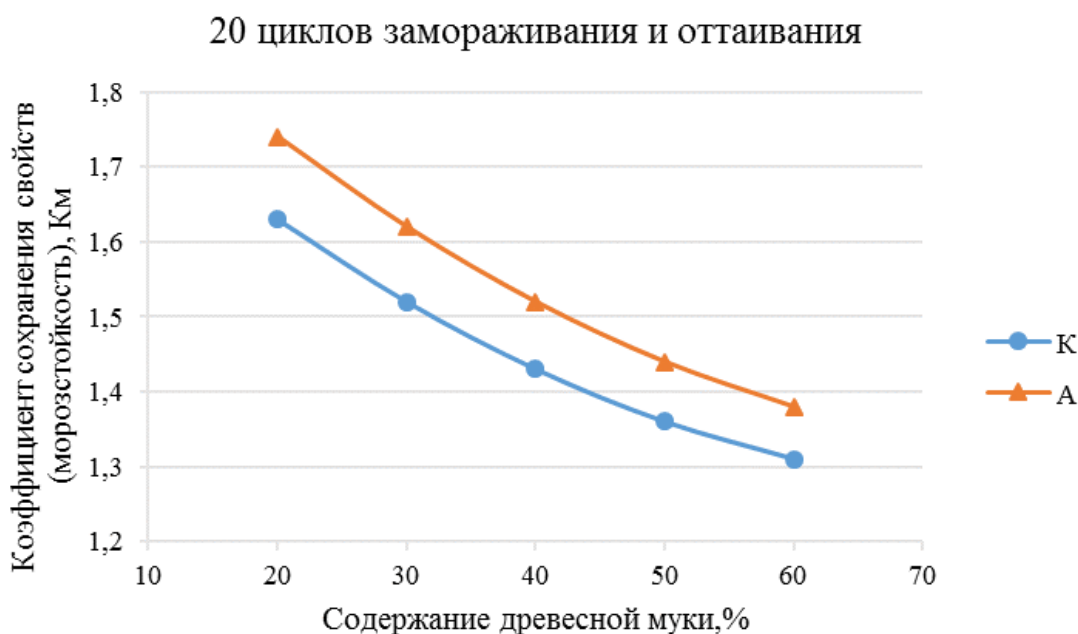
Рисунок 4.30 – Влияние концентрации и предварительной обработки контрольных (К) и ацетилированных (А) составов ДПК на морозостойкость
