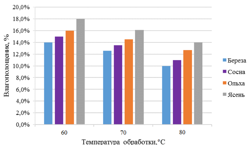
Рисунок 3.9 – Влияние температуры ацетилирования на показатель влагопоглощения для различных пород древесины на 28-е сутки испытаний
