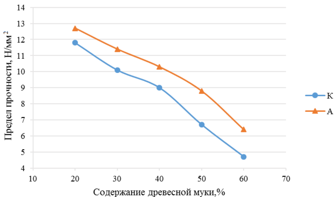
Рисунок 4.20 – Влияние концентрации и предварительной обработки контрольных (К) и ацелированных (А) составов ДПК на предел прочности при растяжении
