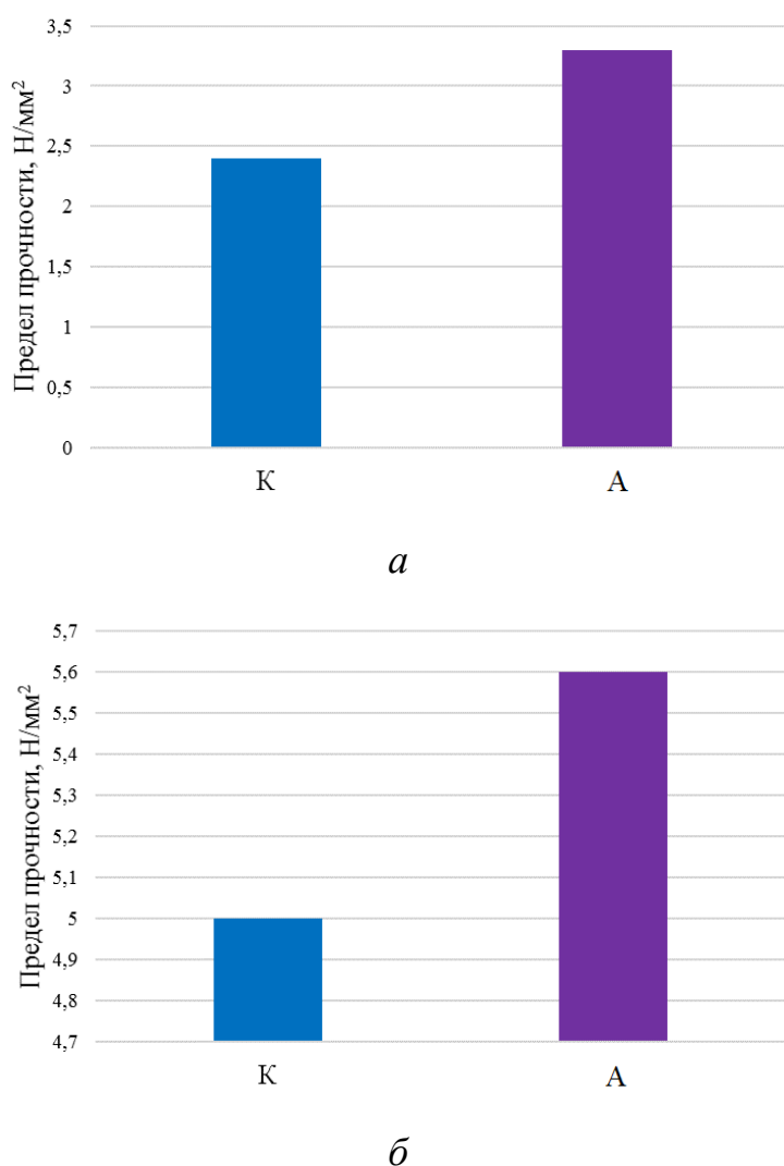
Рисунок 4.17 – Значения предела прочности при изгибе (а) и сдвиге по клеевому шву (б) для контрольных (К) и ацетилованных (А) образцов
