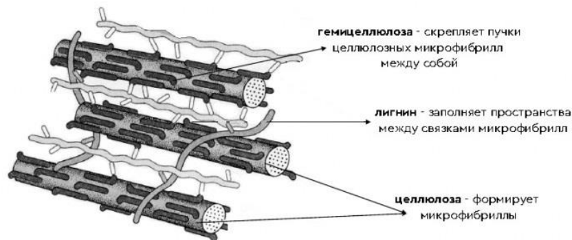
Рисунок 2.1 – Структура клеточной стенки древесины
