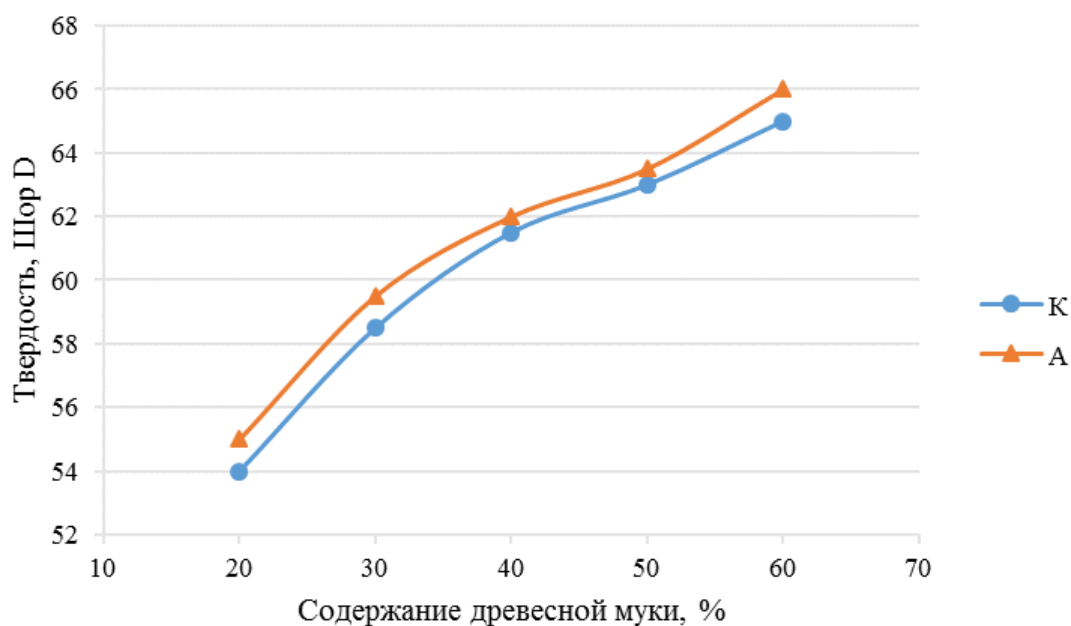
Рисунок 4.19 – Влияние концентрации и предварительной обработки контрольных (К) и ацетилированных (А) составов ДПК на твердость
