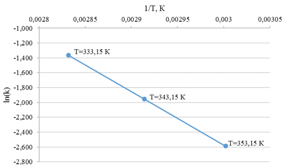
Рисунок 2.6 – Линейная регрессия в координатах \ln(k) от 1/T
