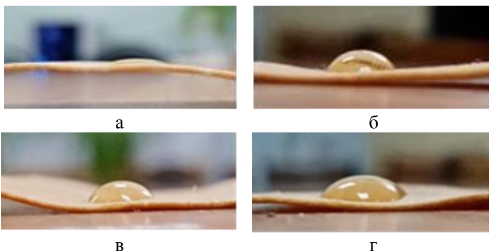
Рисунок 3.4 – Краевые углы смачивания для контрольного образца (а) и ацетилированных образцов в уксусной кислоте при 60°C (б), 70°C (в) и 80°C (г)
