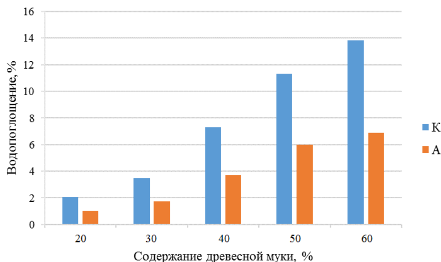
Рисунок 4.28 – Влияние концентрации и предварительной обработки для контрольных (К) и ацетилированных (А) составов ДПК на водопоглощение на 28-е сутки
