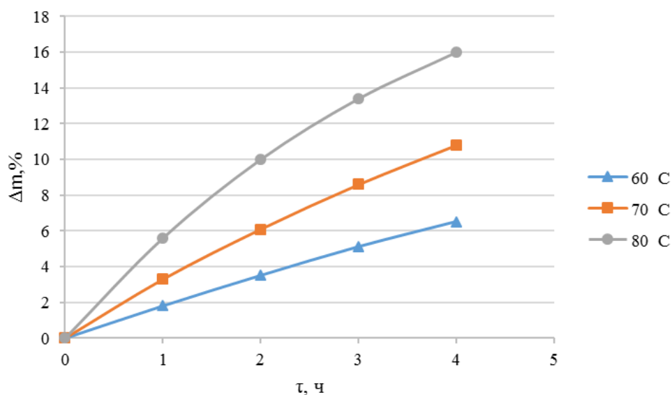
Рисунок 2.4 – Кинетика изменения прироста массы в зависимости от температуры ацетилирования в течение 4 часов
