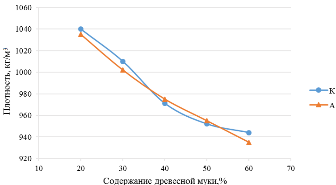
Рисунок 4.18 – Влияние концентрации и предварительной обработки контрольных (К) и ацелированных (А) составов ДПК на плотность
