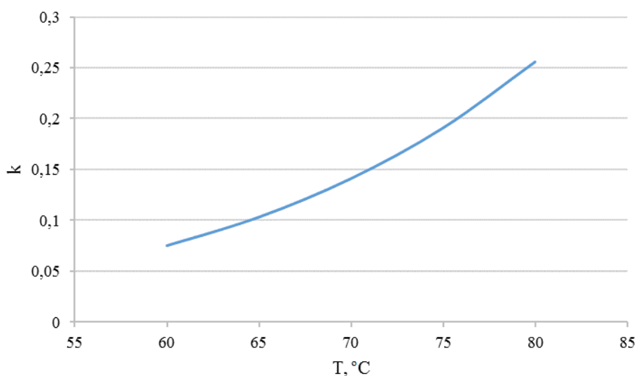
Рисунок 2.5 – Зависимость константы скорости химической реакции от температуры обработки
