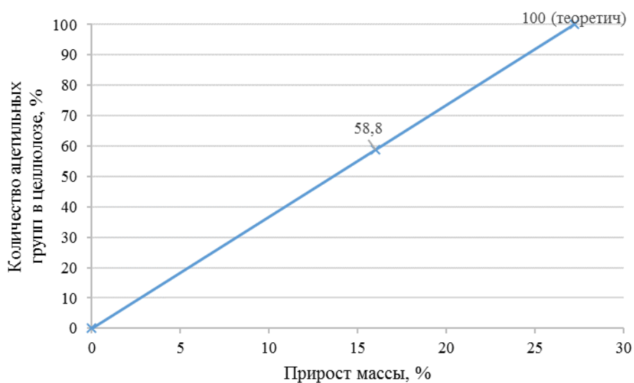
Рисунок 2.7 – Линейная зависимость количества ацетильных групп в целлюлозе в зависимости от прироста массы
