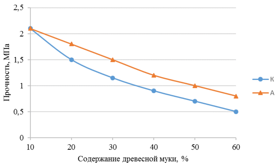
Рисунок 5.5 – Зависимость усилия разрыва для ацетилированного (А) и контрольного (К) составов древесно-полимерного композита
