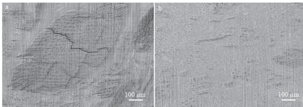
Рисунок 1.7 – Сканирующие электронные микрофотографии древесно-пластиковых композитов, формованных под давлением, с пропионат-ацетатом целлюлозы в качестве матрицы: (а) с немодифицированным древесным наполнителем; (б) с ацелированным древесным наполнителем
