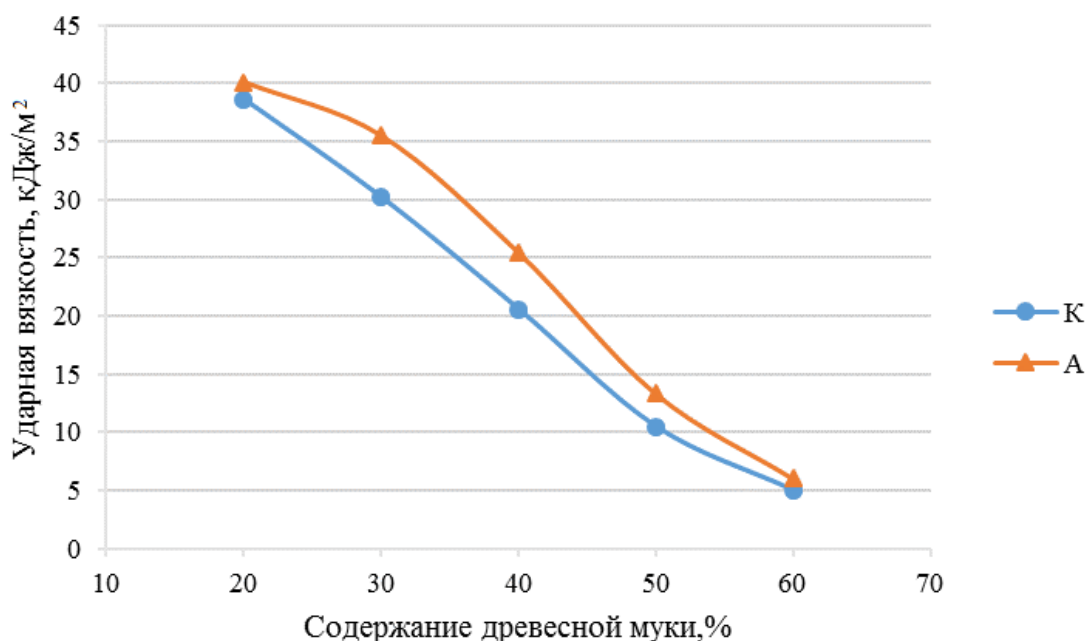
Рисунок 4.22 – Влияние концентрации и предварительной обработки контрольных (К) и ацелированных (А) составов ДПК на ударную вязкость
