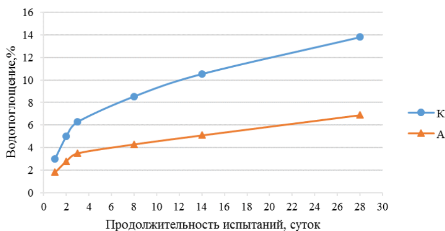
Рисунок 4.27 – Водопоглощение ДПК с 60 %-м содержанием наполнителя
